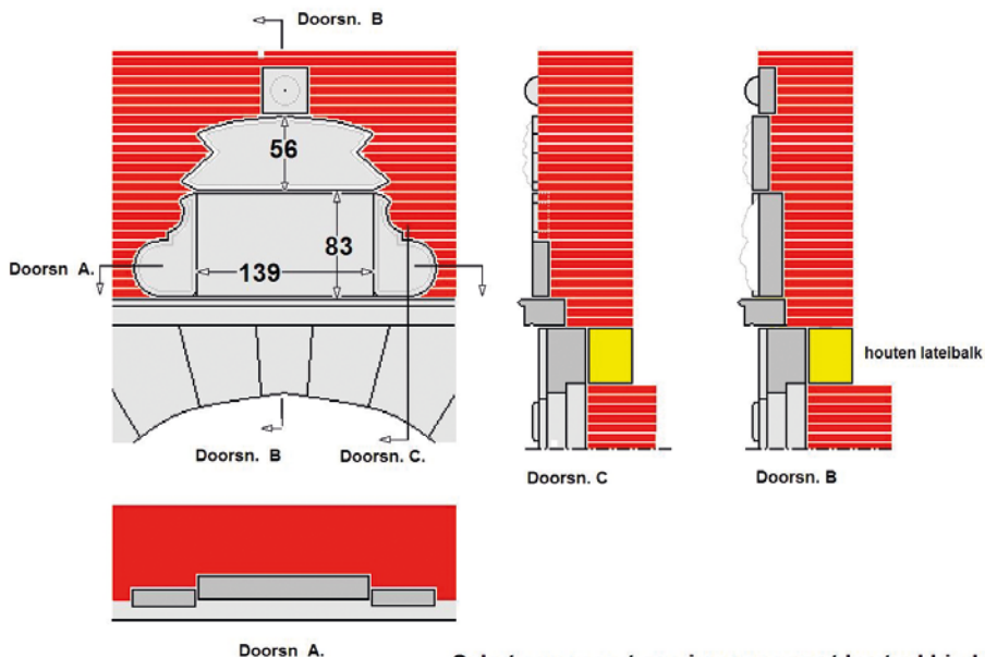
Schets wapenstein ingangspoort kasteel Limbricht
